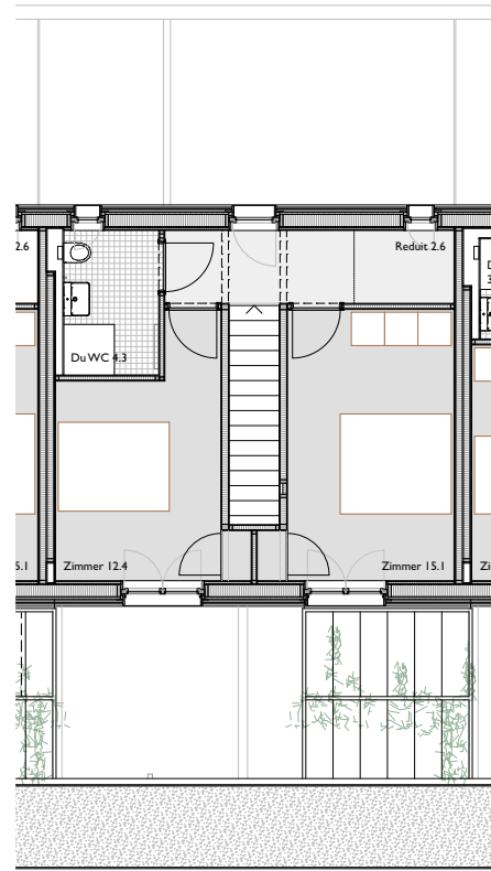
2.OG
