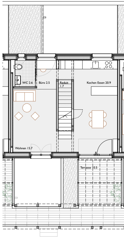
1.OG
