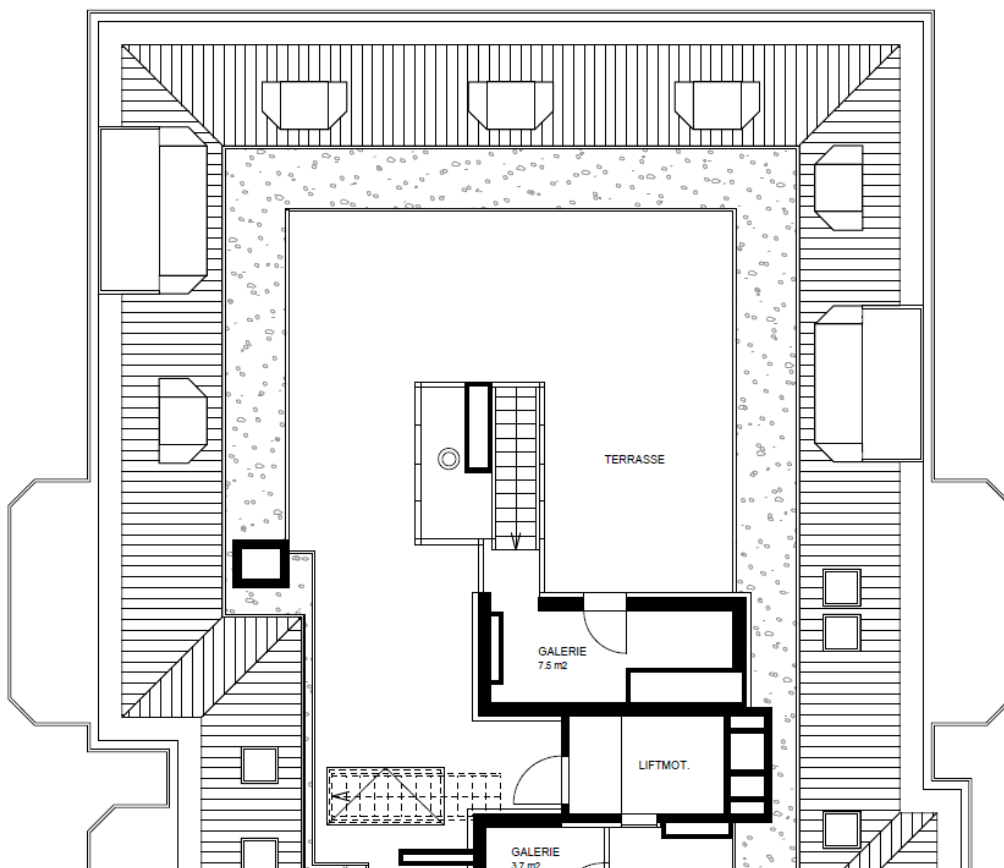
Dachterrasse
