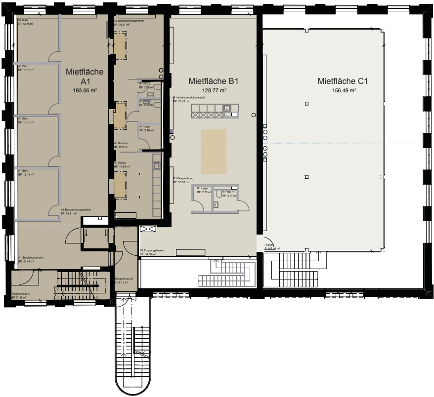
1. Obergeschoss
