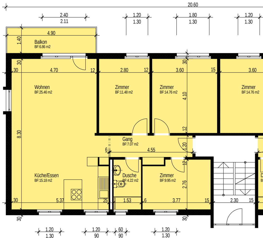
Grundriss
