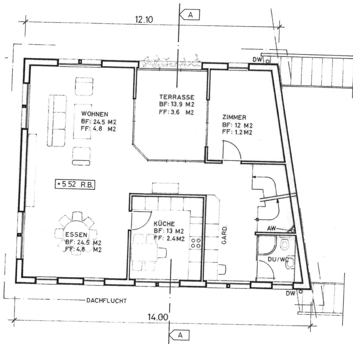
GRUNDRISS 2. OBERGESCHOSS
