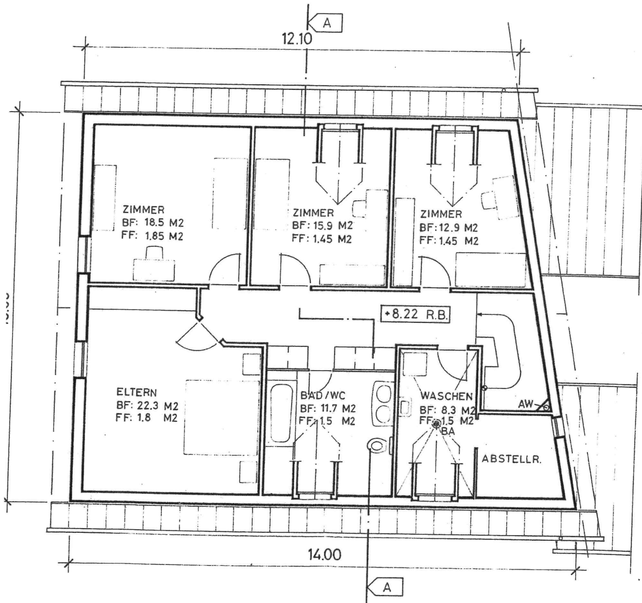
GRUNDRISS DACHGESCHOSS
