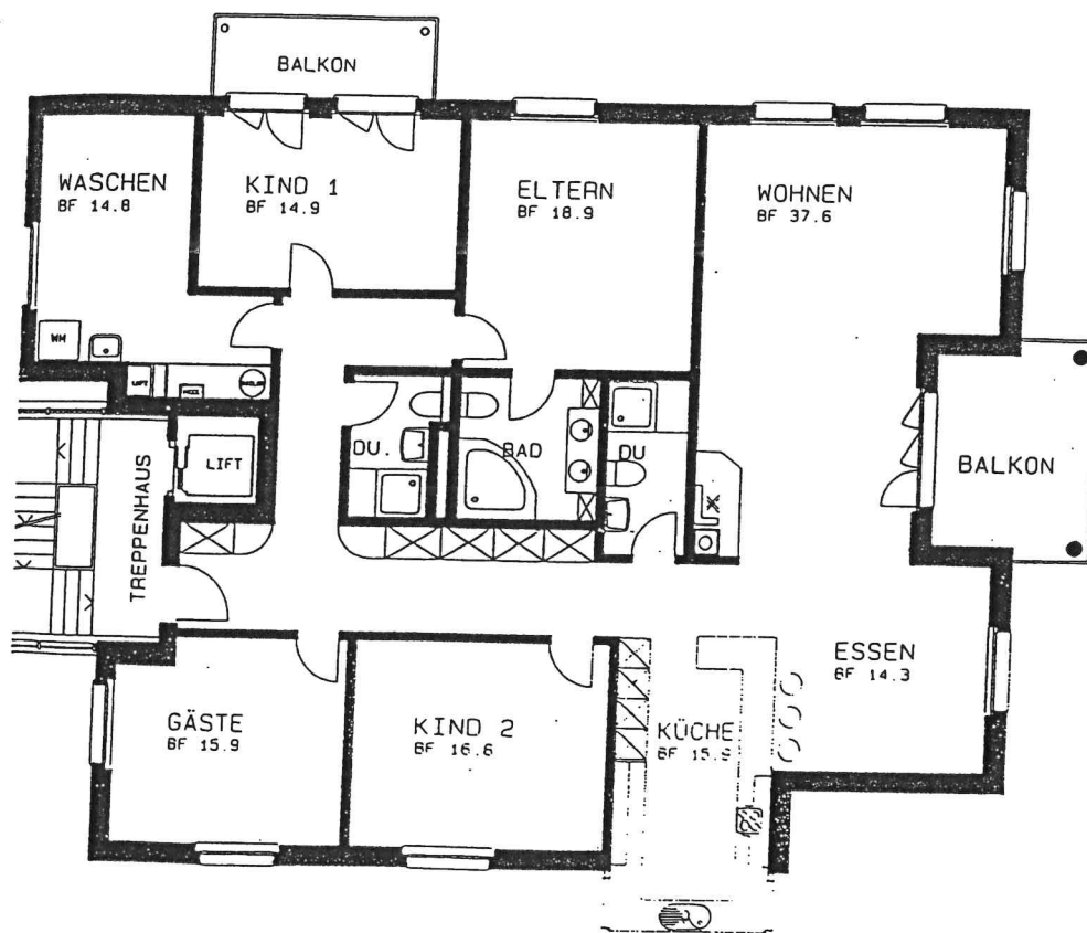
1. + 2. OBERGESCHOSS
