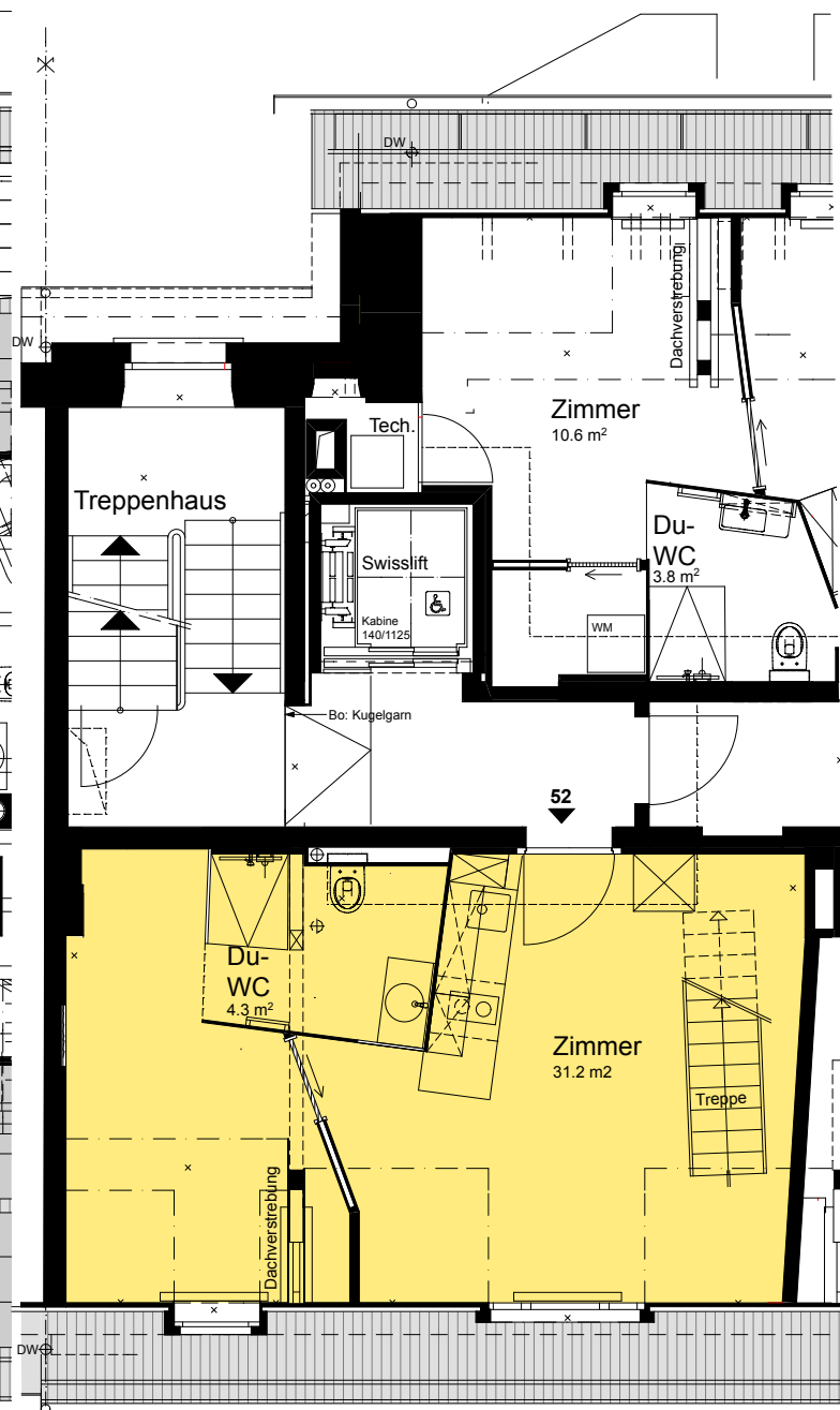
5. Obergeschoss
