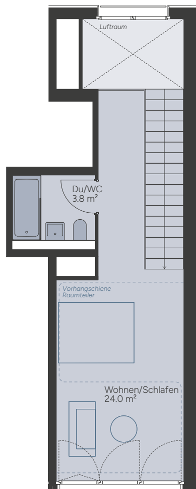
1. Obergeschoss
