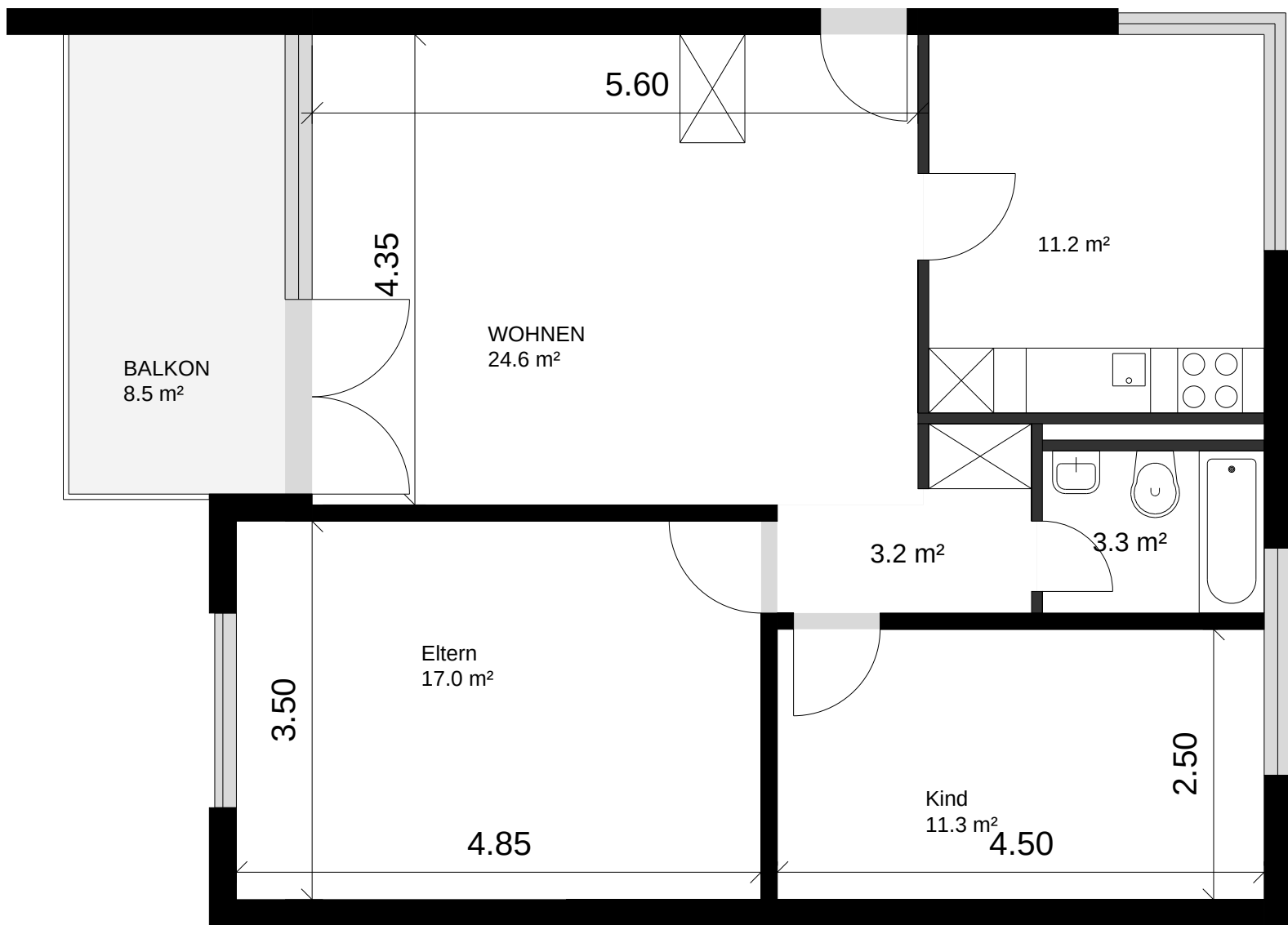
Grundrissplan
