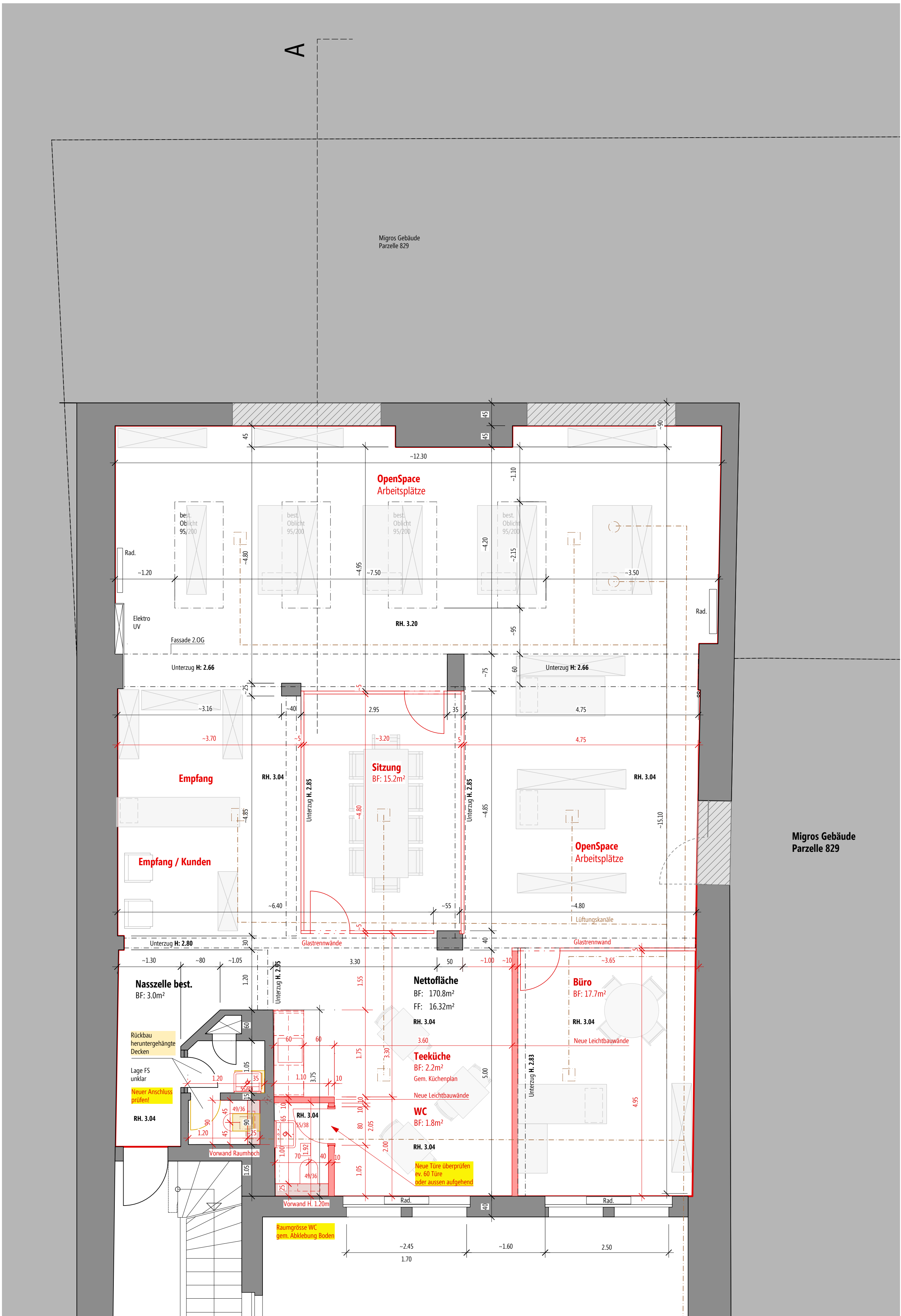
1. OG Ausschnitt / Umnutzung Mst. 1:50
