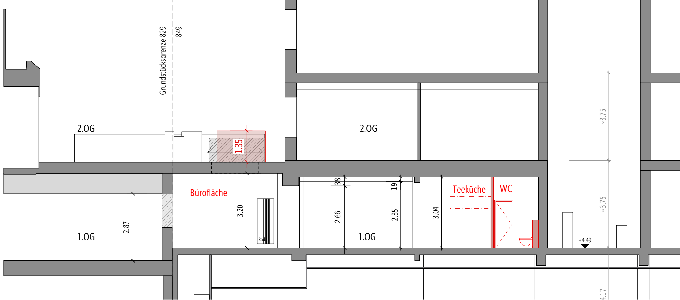
Längsschnitt Ausschnitt Mst. 1:100
