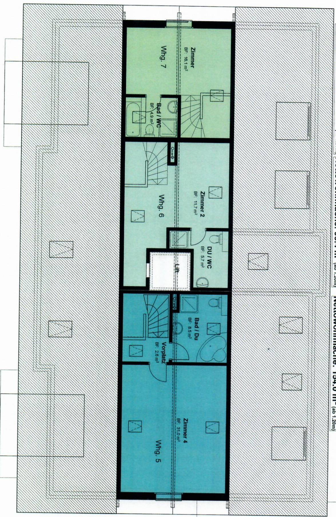
Dachgeschoss 1:10
