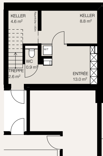
UNTERGESCHOSS
