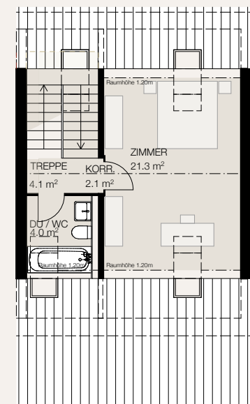
1. OBERGESCHOSS
