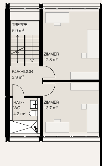
1. OBERGESCHOSS
