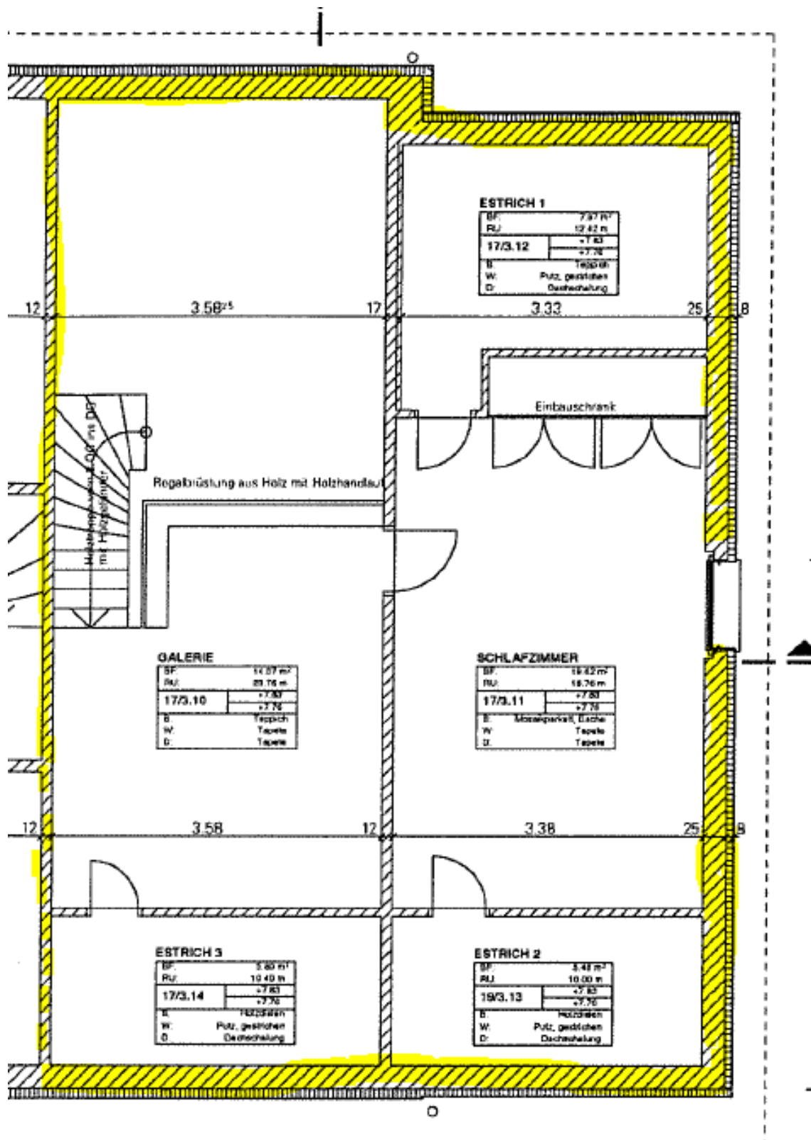
5.5-Zimmer Maisonettewohnung im 2. OG / 2. Geschoss
