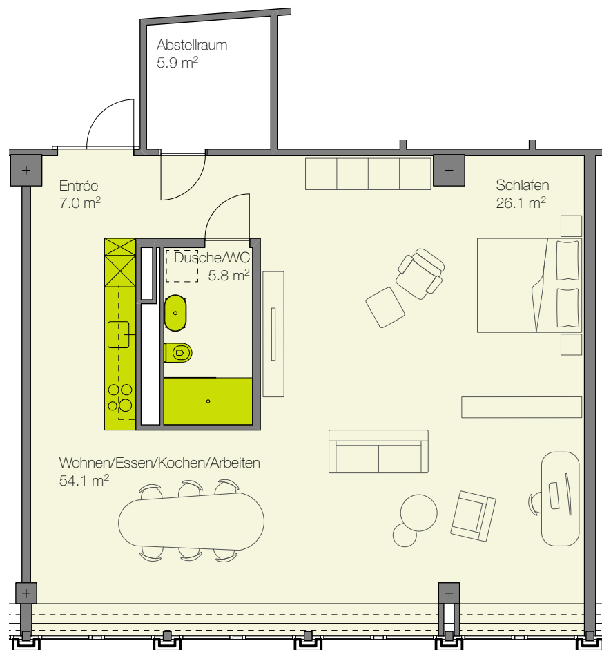
Grundriss 2. Obergeschoss Mst. 1:100
