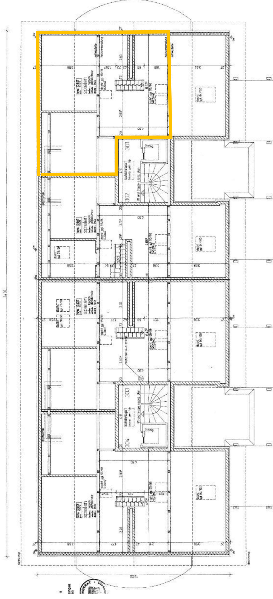
Galeriegeschoss Block a + b
