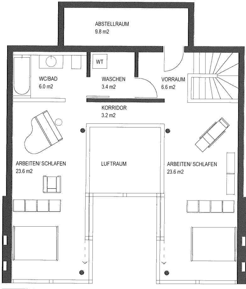
1. Obergeschoss
