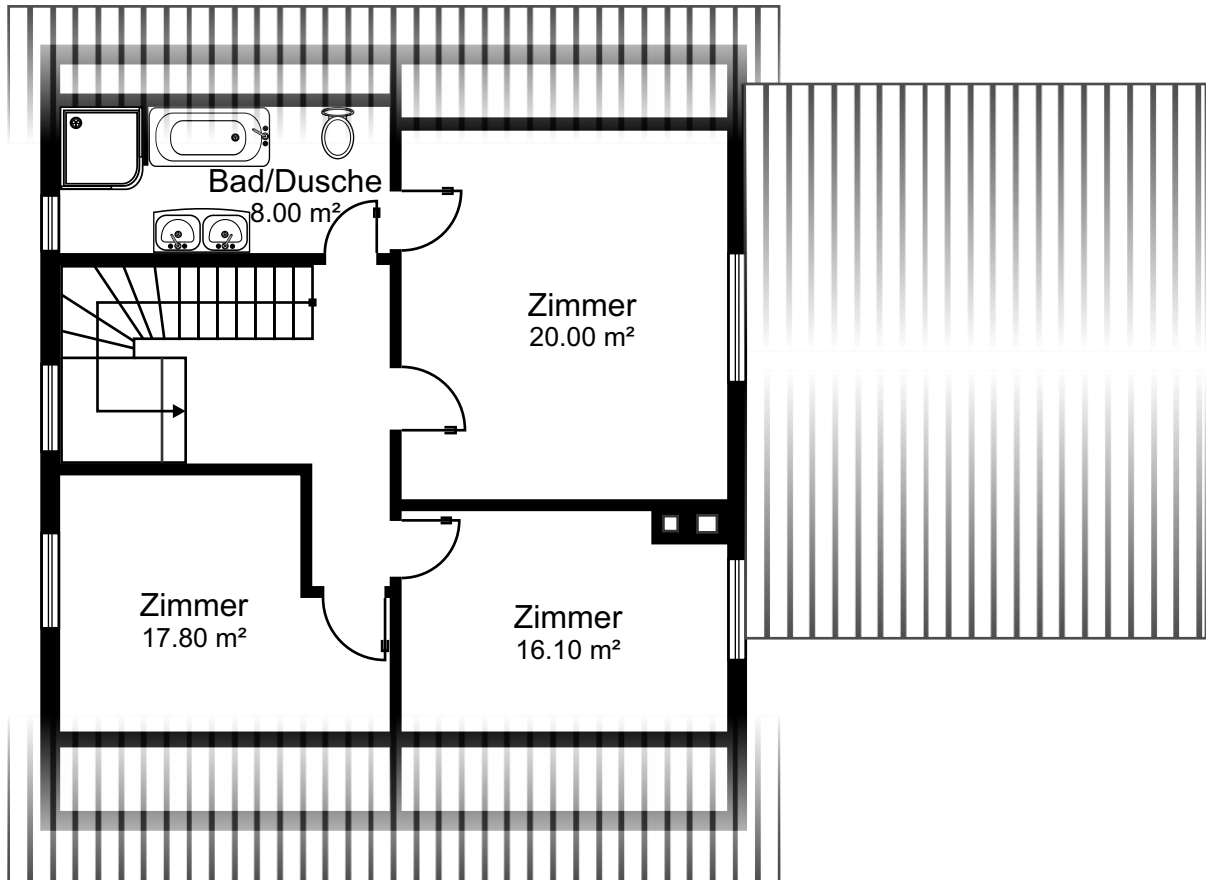
1. Obergeschoss
