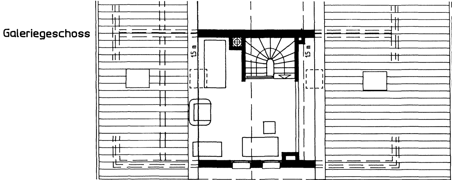
Grundrisse
