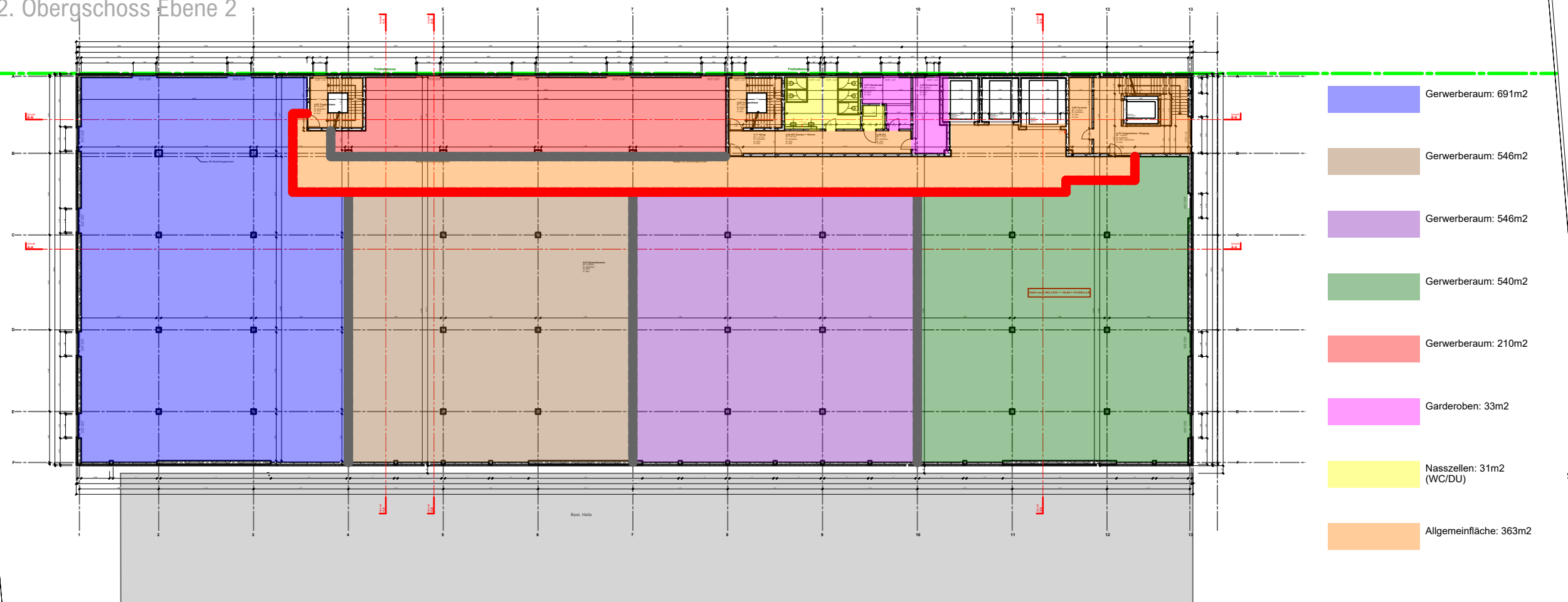
2. Obergeschoss Ebene 1
