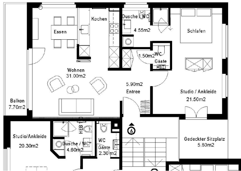
Grundriss 2.5-Zimmer Wohnung im 1. OG
