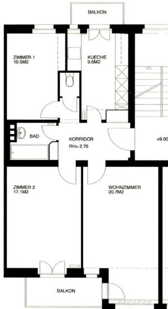
3. OBERGESCHOSS
