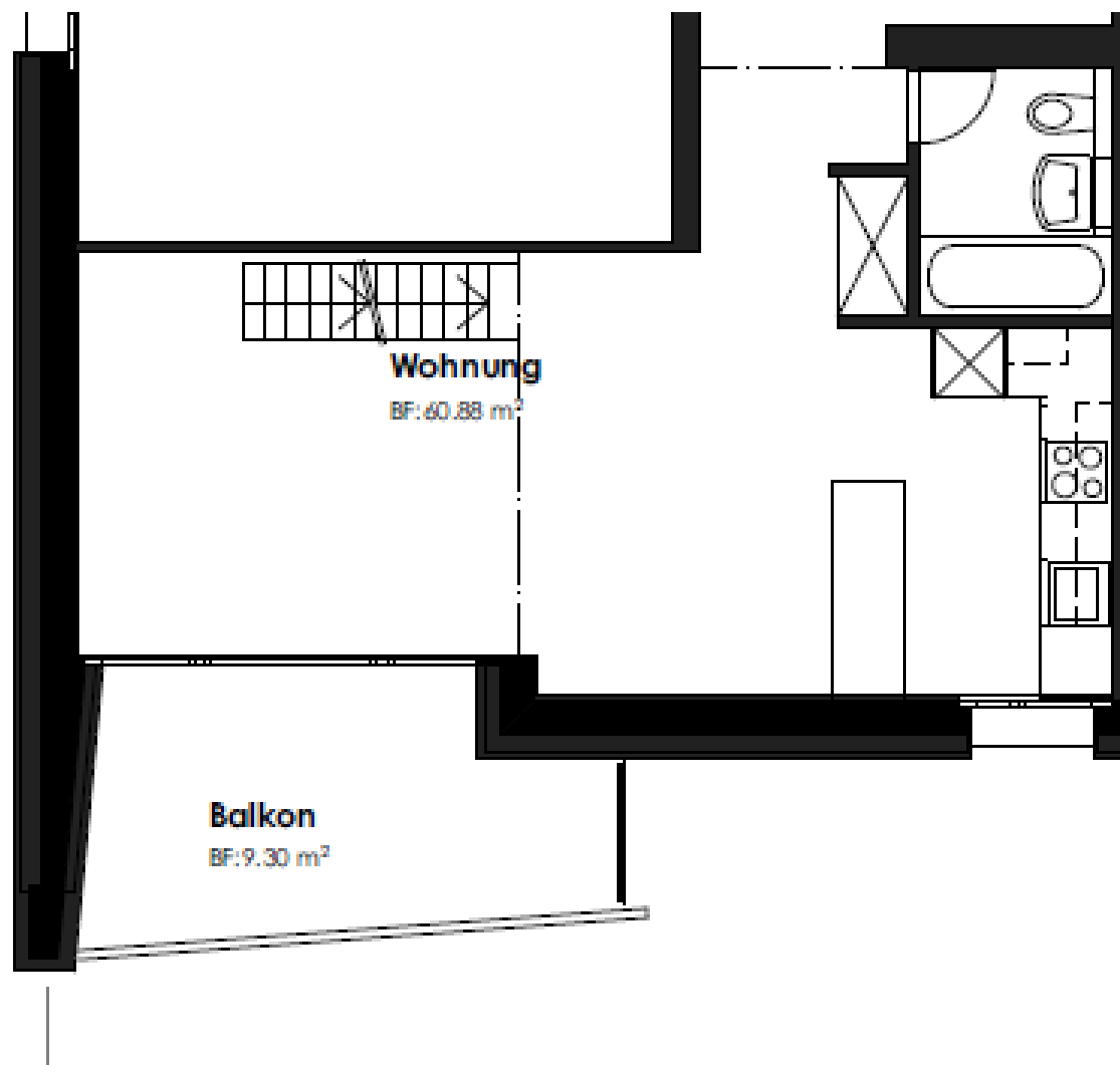
Grundriss 01311.01.1203 2.5 Zimmer-Maisonette im 2.OG, untere Etage
