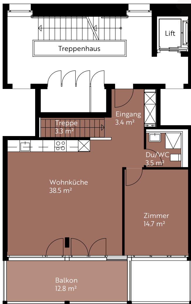
5. Obergeschoss
