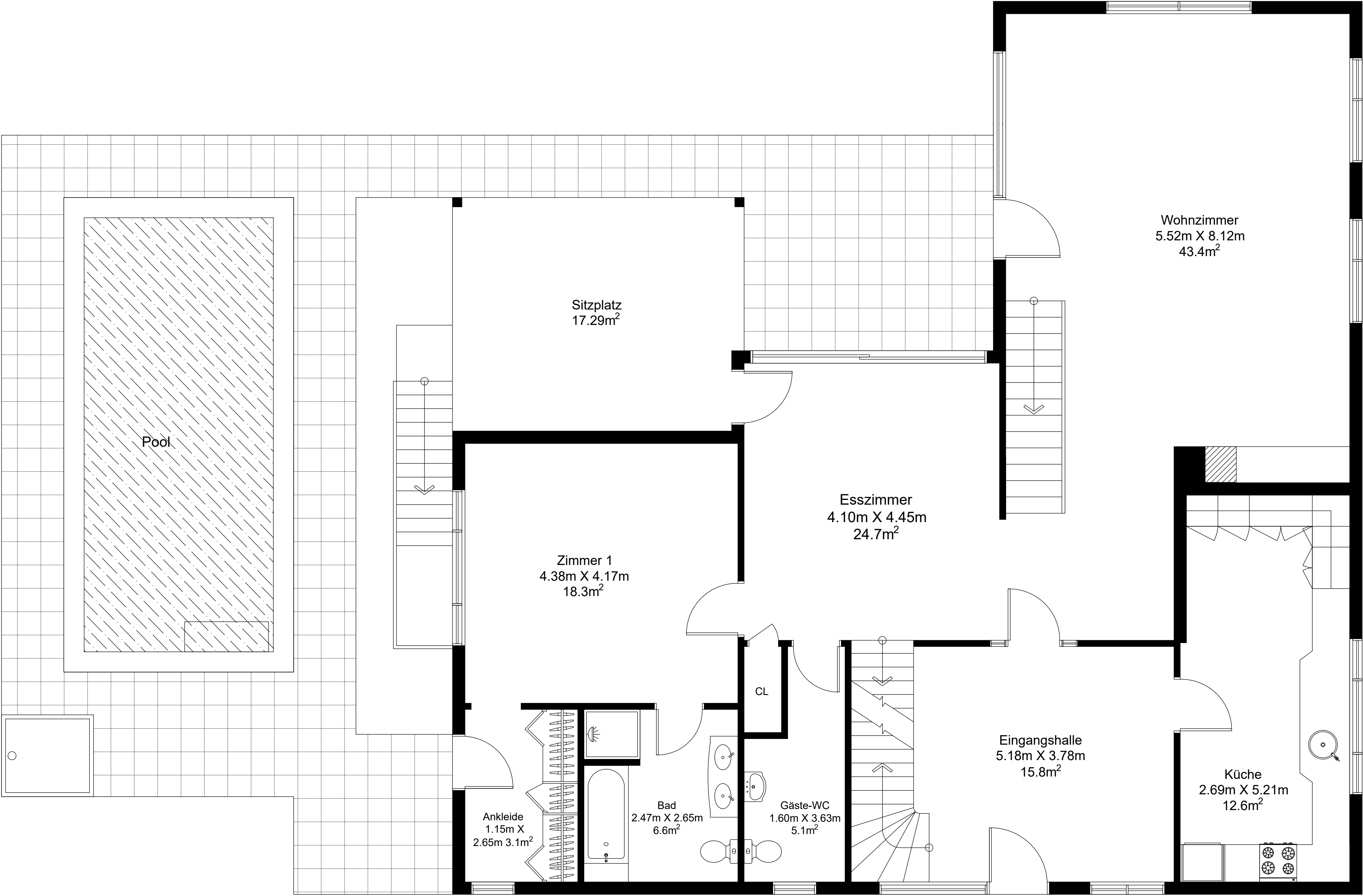
Erdgeschoss
