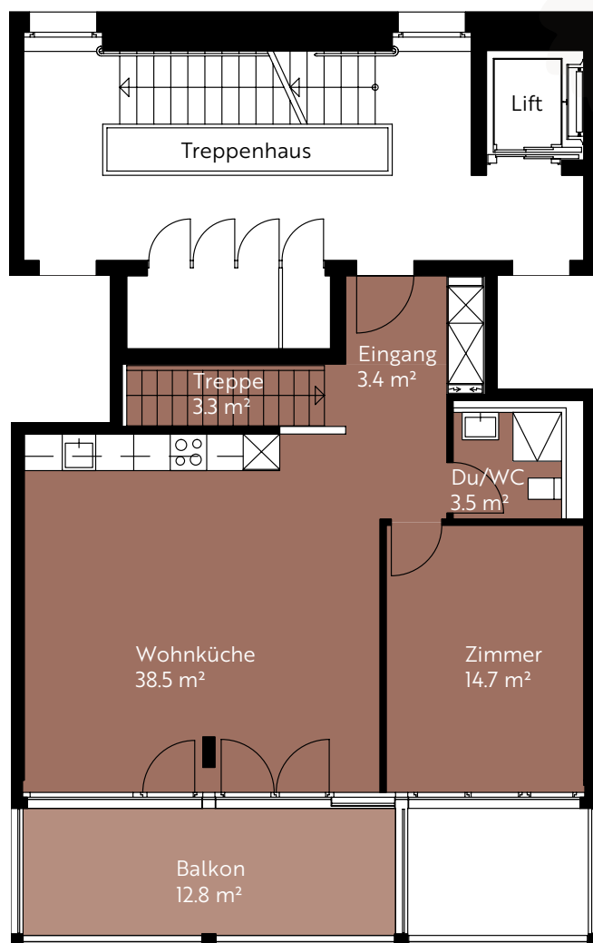
5. Obergeschoss
