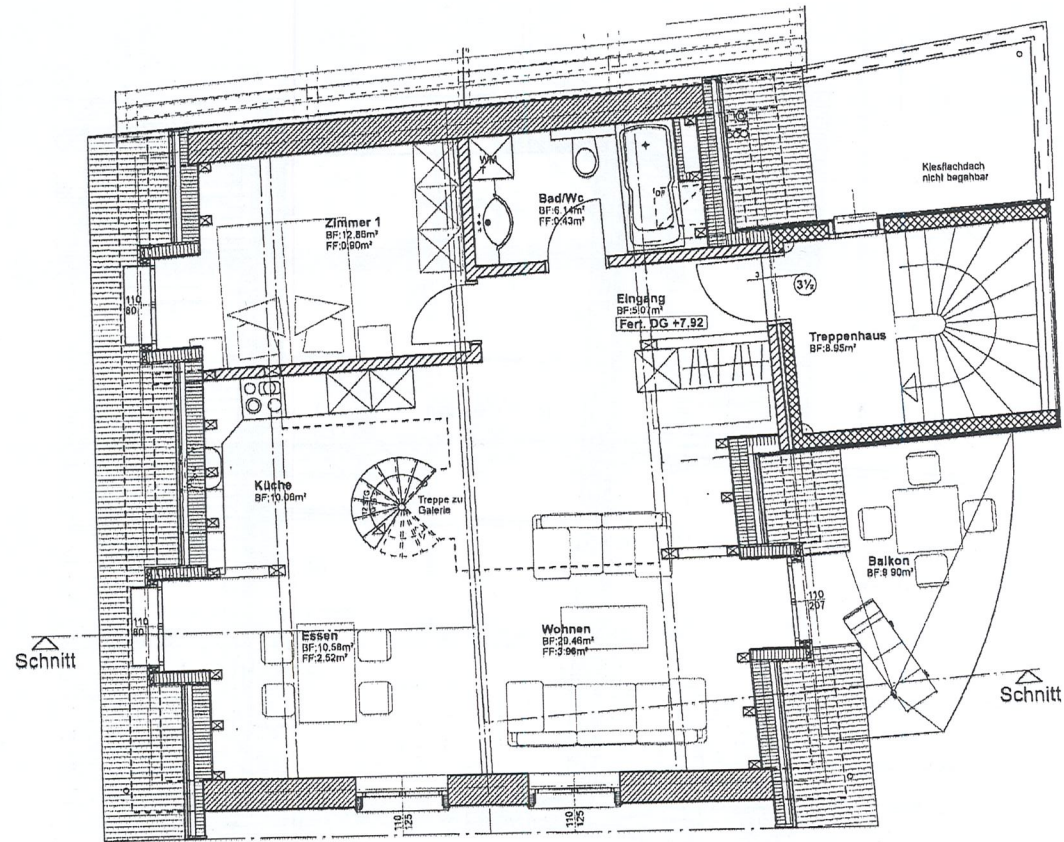
Dachgeschoss
