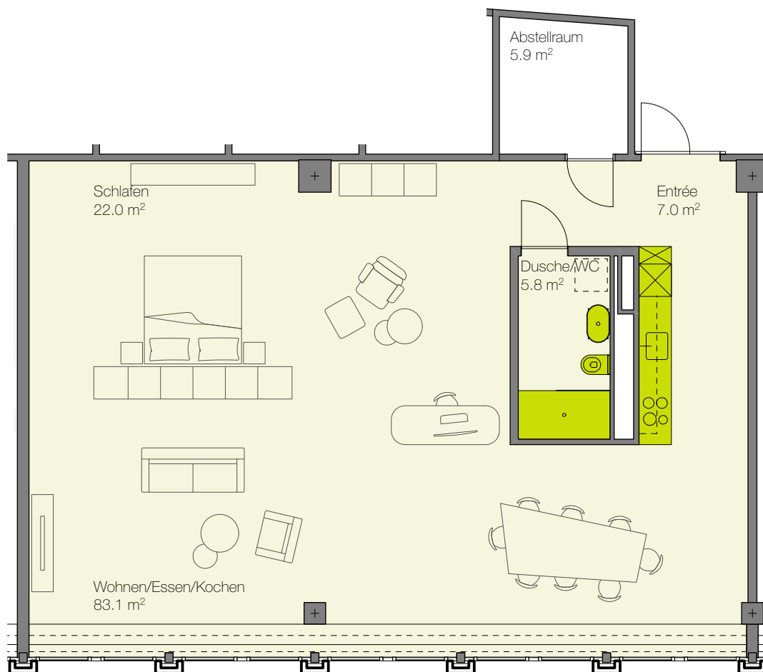
Grundriss 3. Obergeschoss Mst. 1:100
