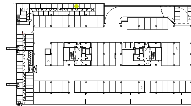
Grundriss 2. Untergeschoss Mst. 1:1000
