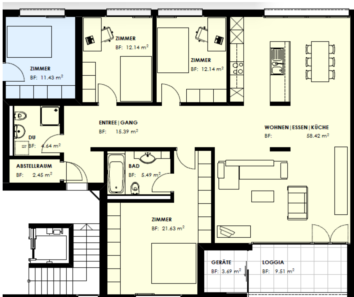
4.5 Zimmerwohnung 3. OG _ Espenmoosstrasse 10 9008 St. Gallen
