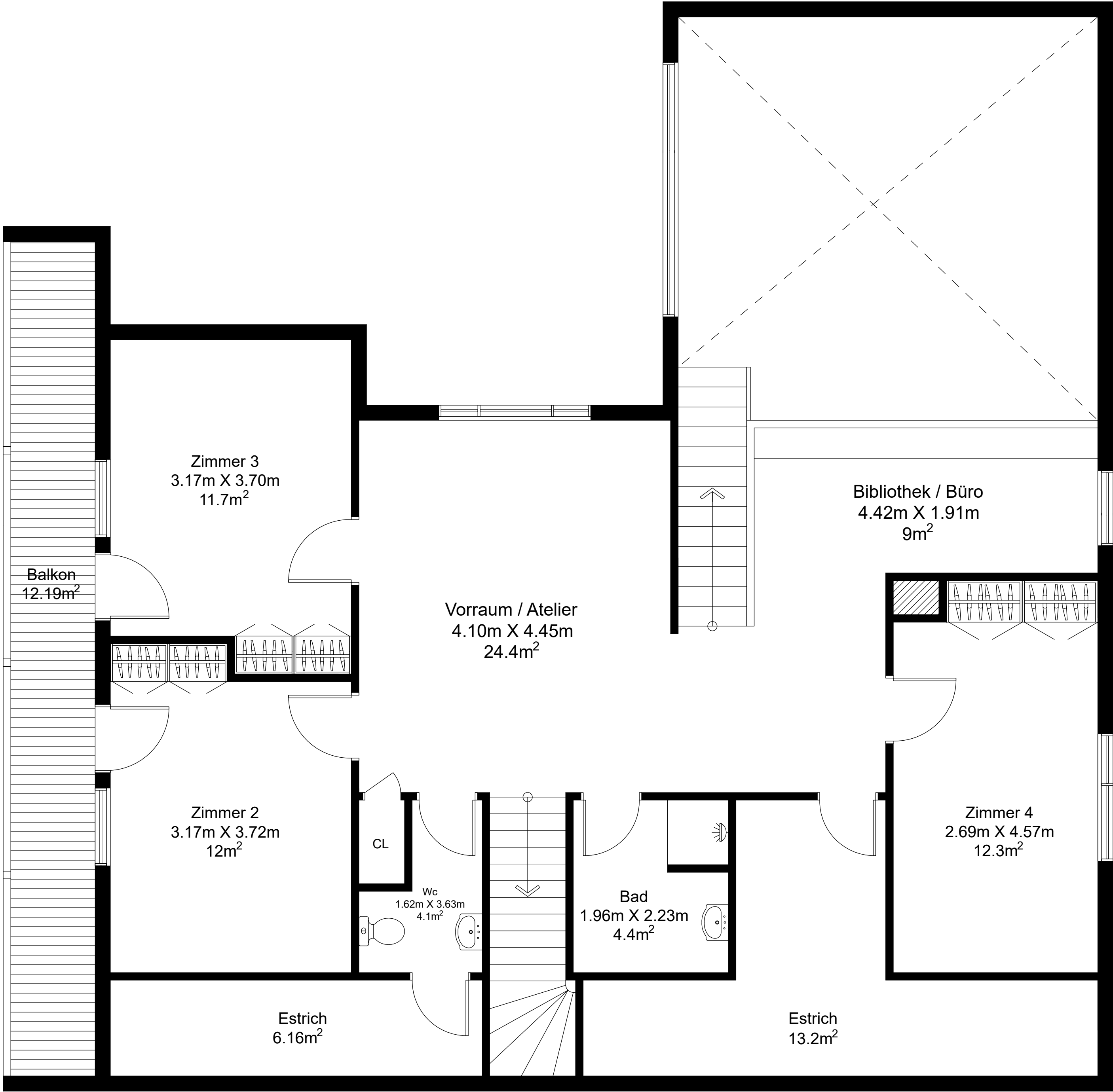
Obergeschoss
