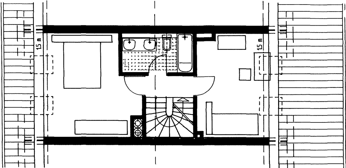
Dachgeschoss
