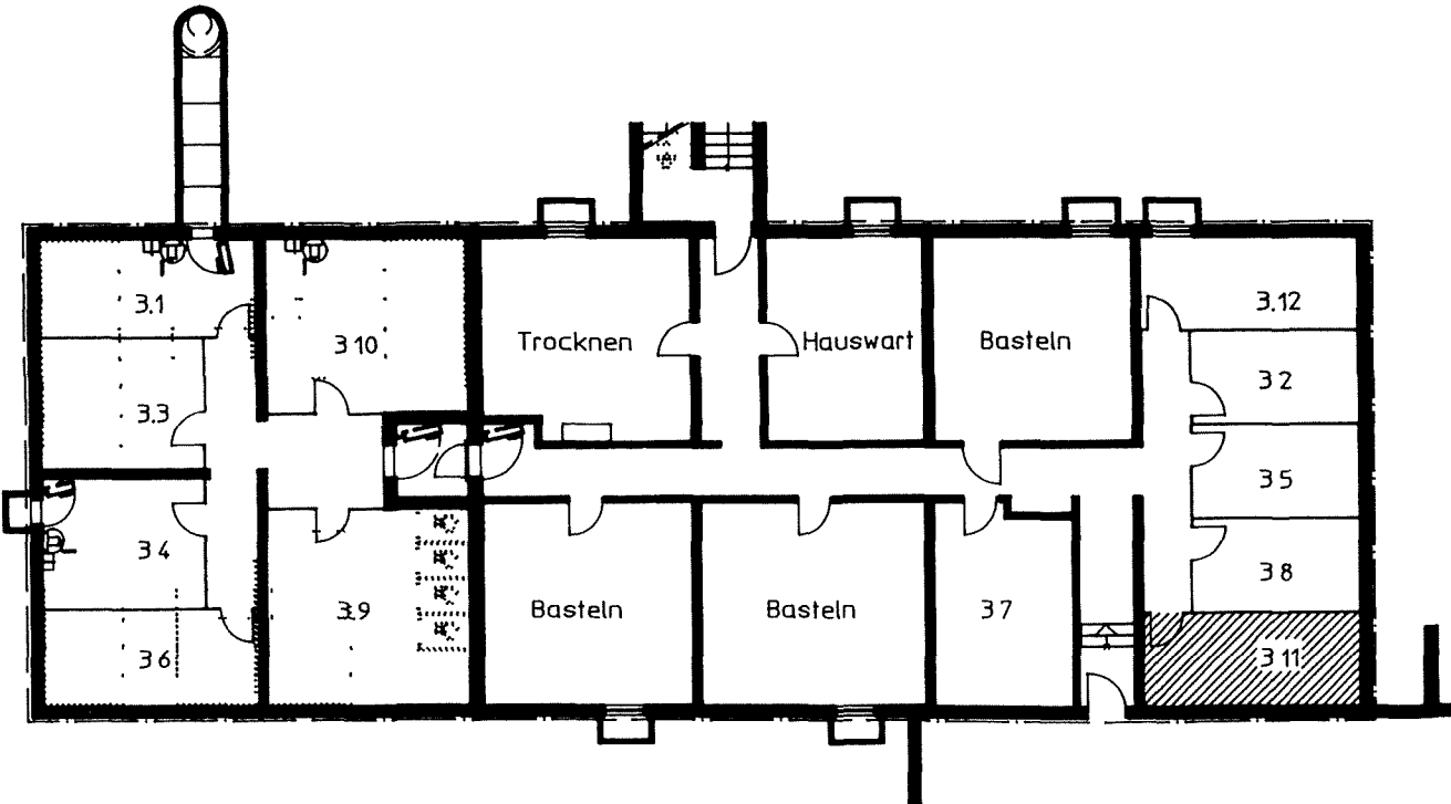
Keller Haus 3
