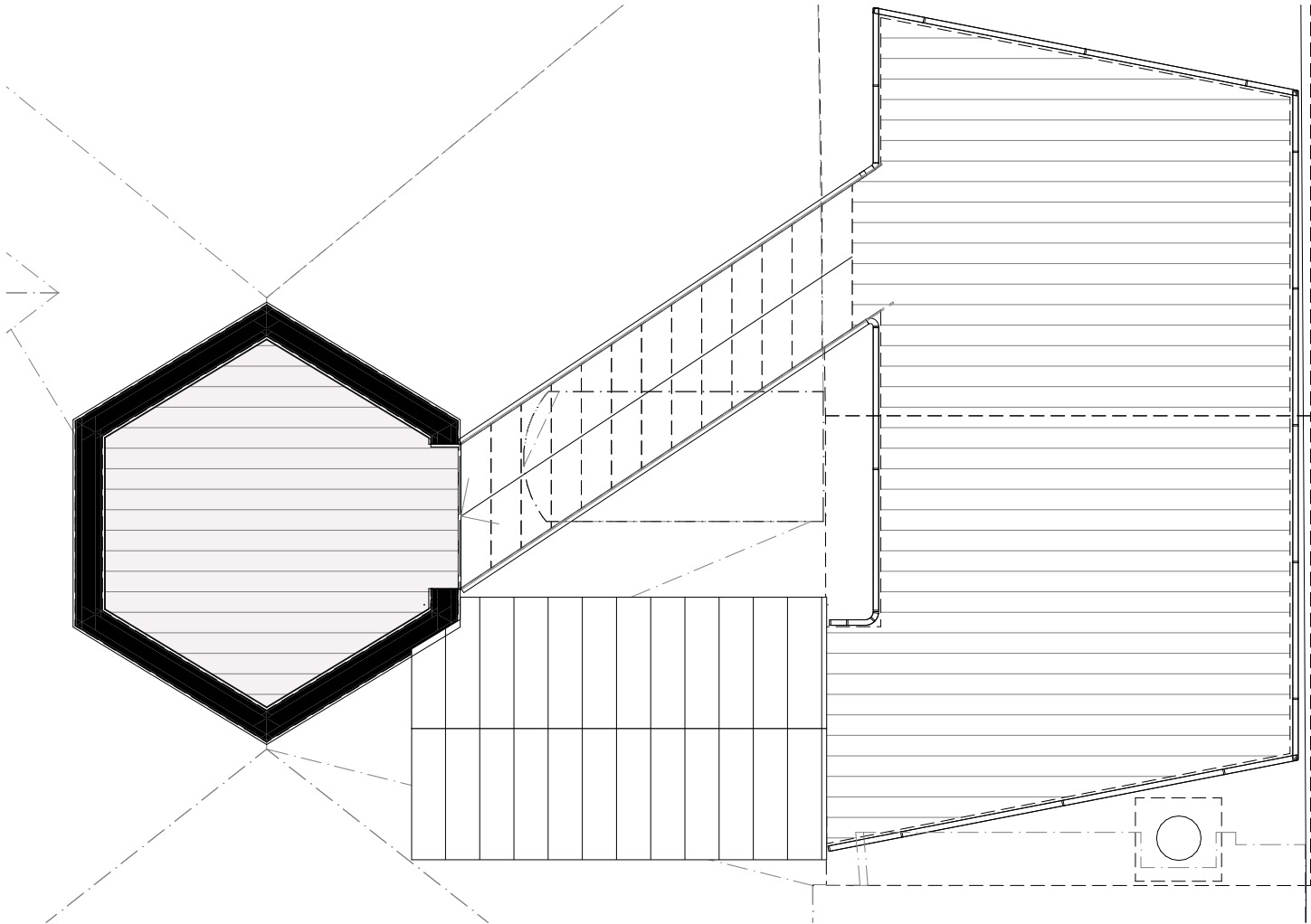
Dachaufsicht 1:50
