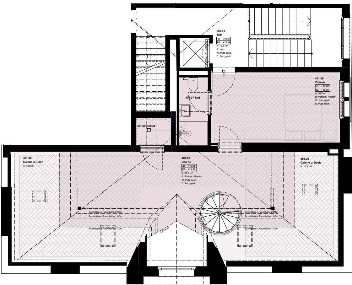
DG 1 1:100
