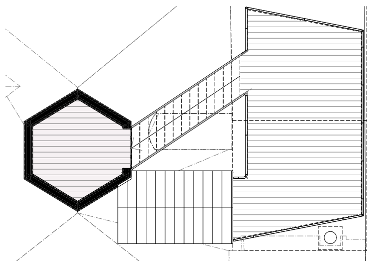
Dachaufsicht 1:100
