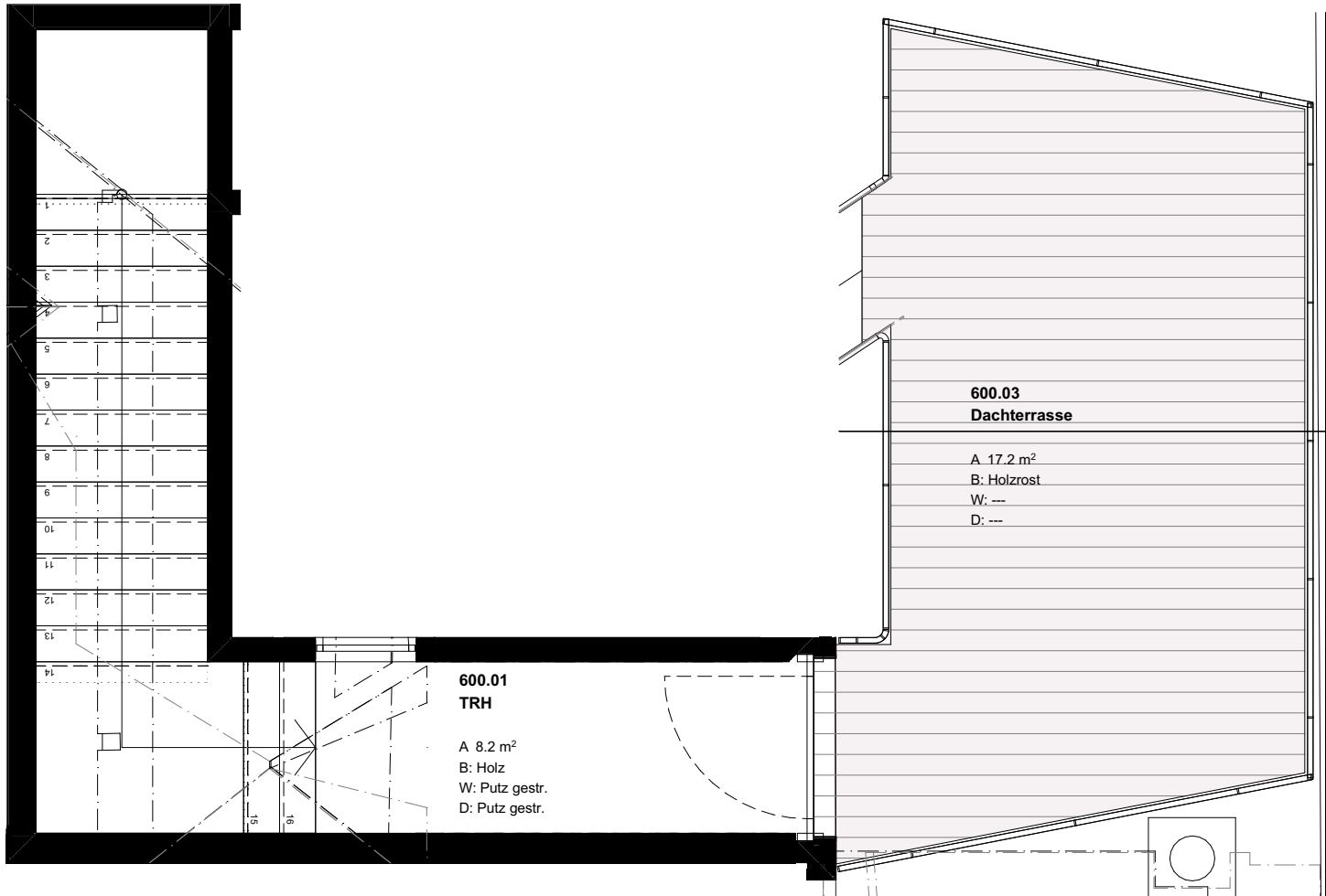
DG 2 1:50
