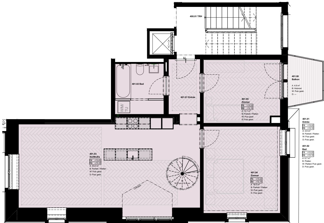
OG 4 1:100
