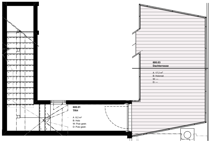
DG 2 1:100
