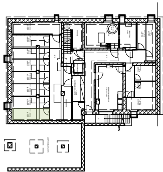
UG mit Kellerabteil Mst 1:100
