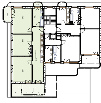
1. OG Mst 1:100
