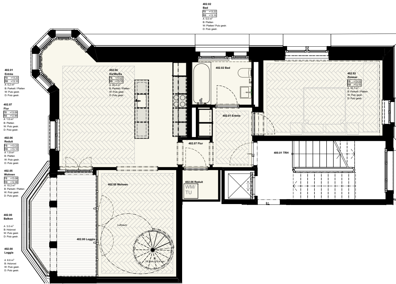
OG 4 1:100
