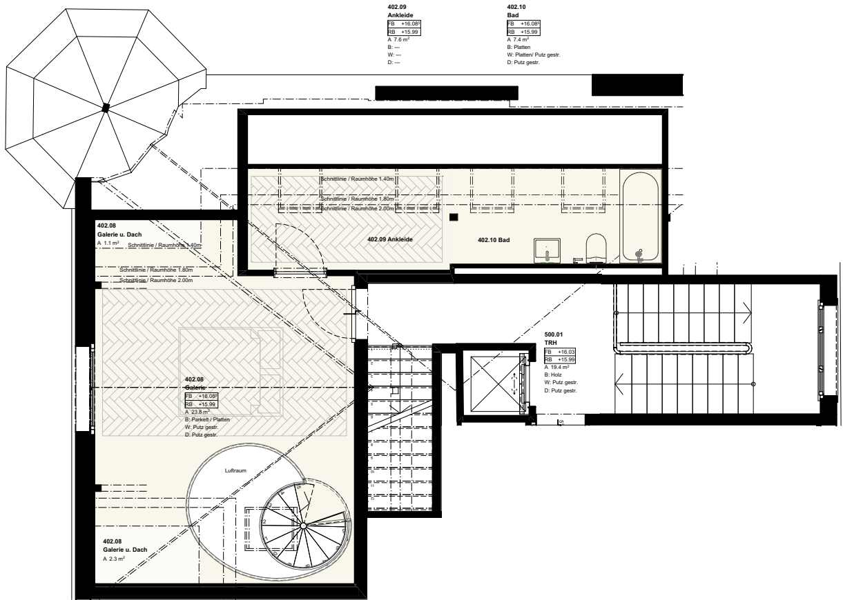
DG 1 1:100
