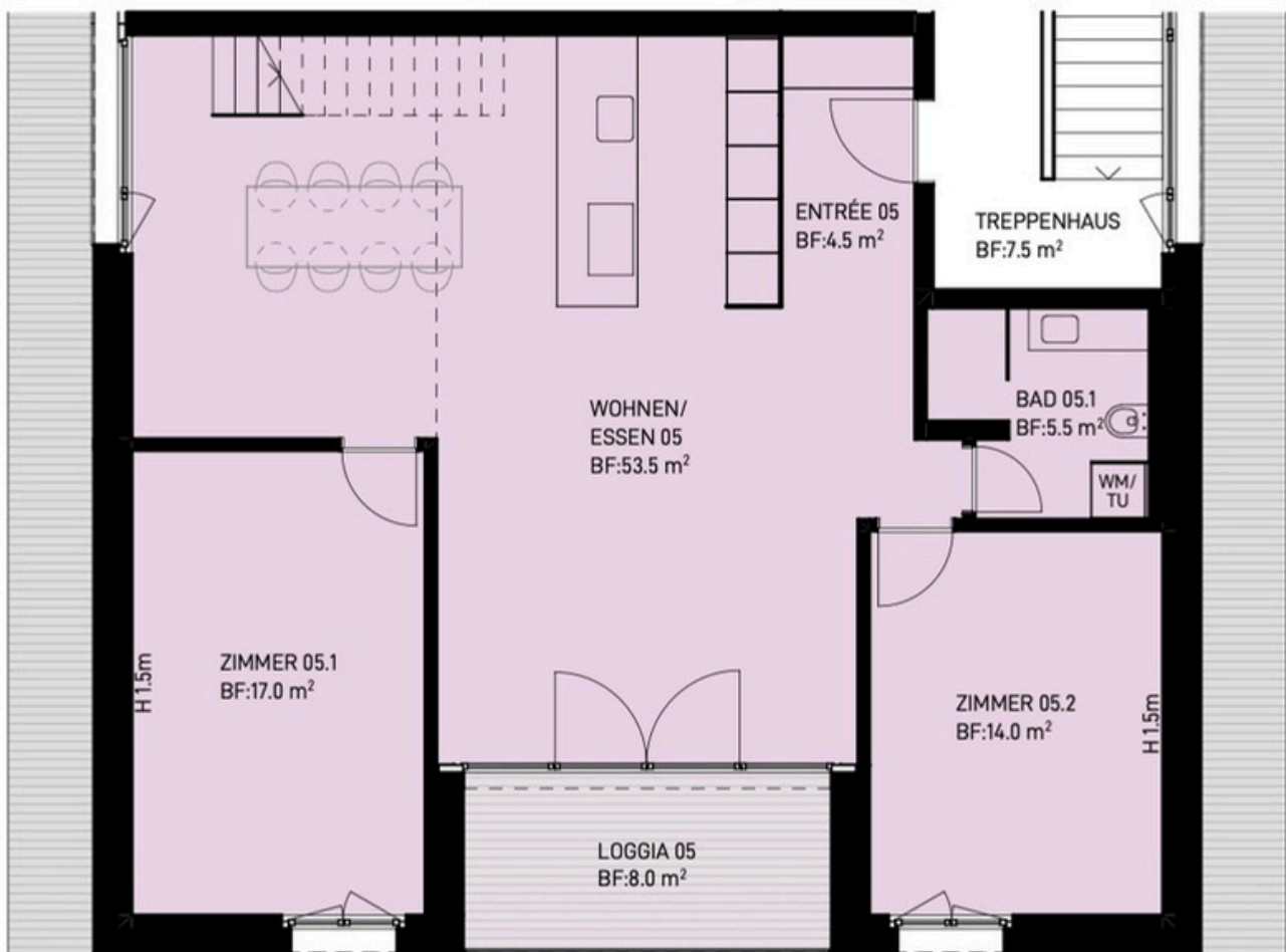
1. DACHGESCHOSS
